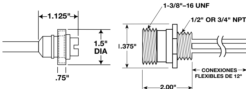
VISTA FRONTAL DEL ENSAMBLE DE ENCHUFE HEMBRA
